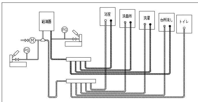
水圧検査概略図
