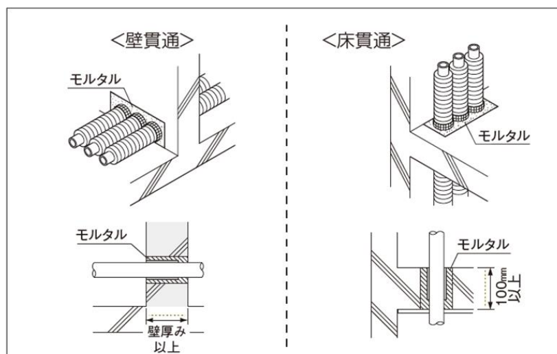
図－26 埋め戻し
