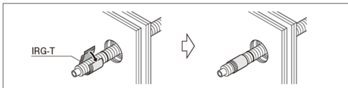
図-30 耐火プラグの巻き付け
