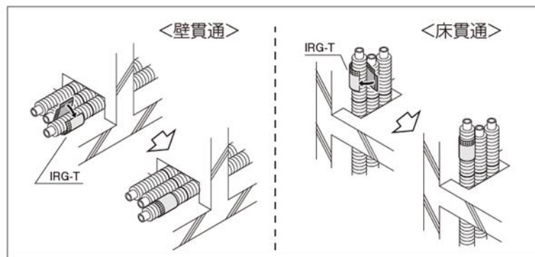
図－24 耐火テープの巻き付け
