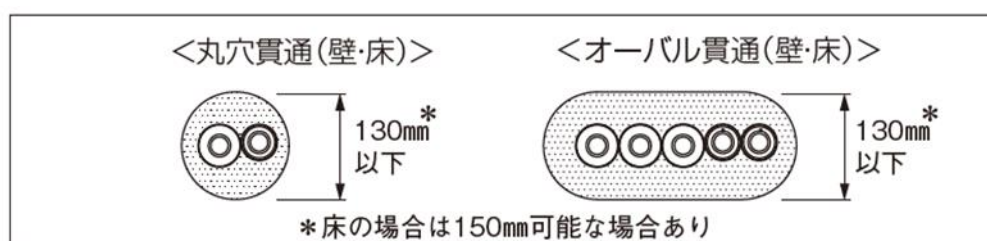
図-21 丸穴貫通の場合
