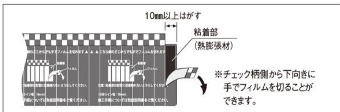
図-29 耐火テープの長さ調整
