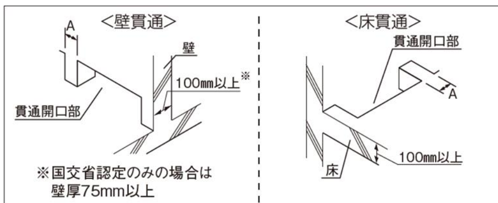
図-19 貫通開口部の設定
