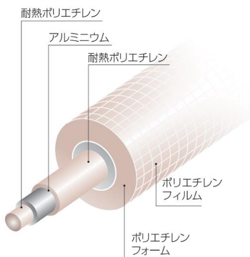
図-14 管の特長
