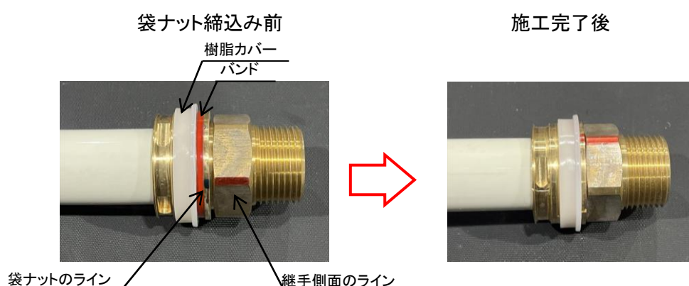
図－5 施工完了確認機構
