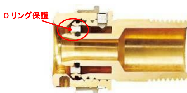
図ー9 Oリングの抜け出し防止スポンジ
