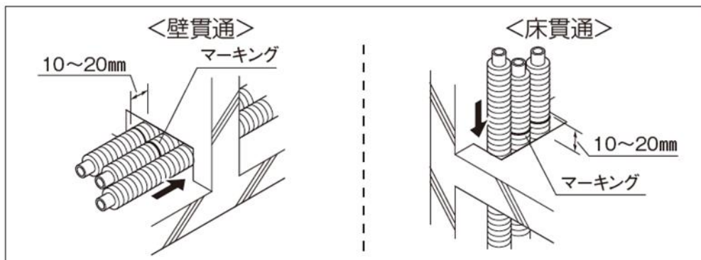
図－22 配管の設置
