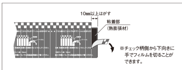
図－23 耐火テープの長さ調整
