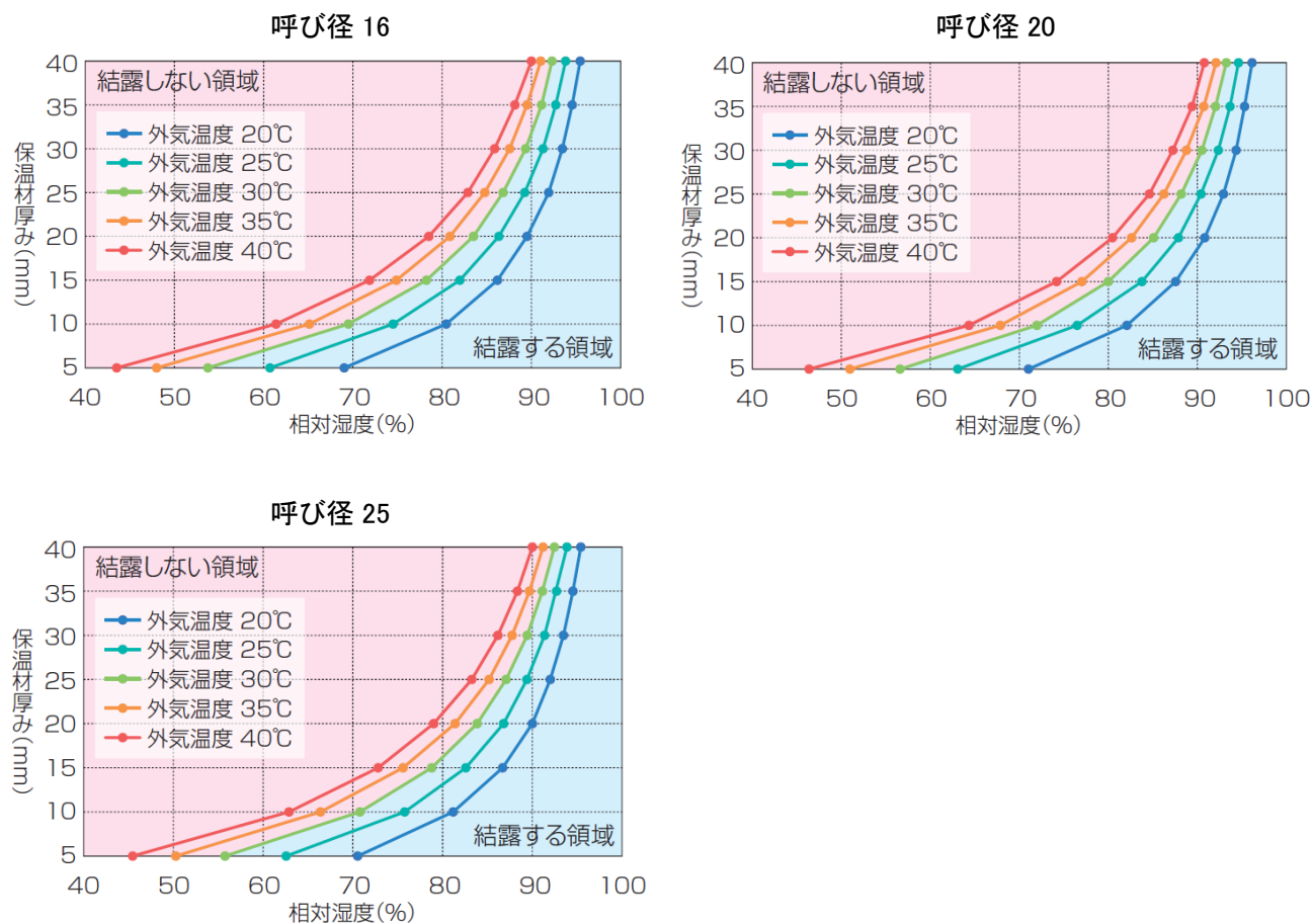
図-17 水温 7°Cによる外気温と保温材厚さによる結露条件
