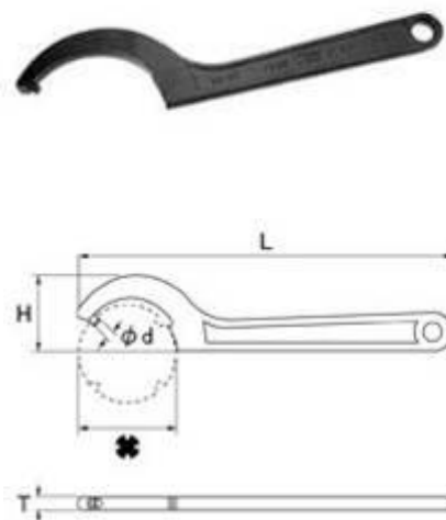
図－11 引掛ピンスパナ詳細
