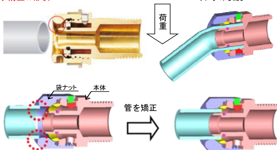
図-1 継手端面 R 形状
