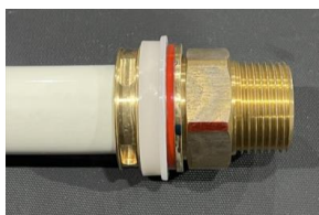
手順①管挿入
