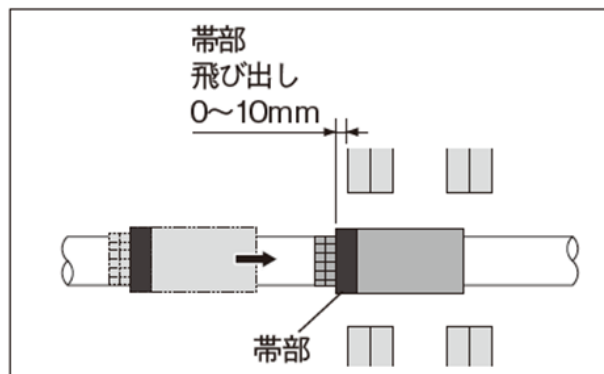
図-31 耐火プラグのスライド
