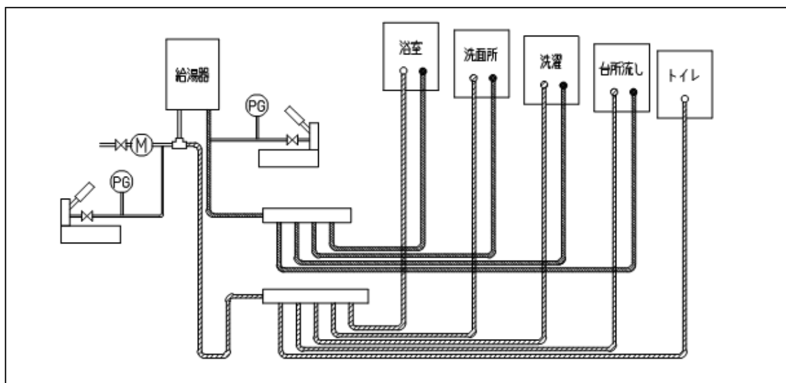
図-18 水圧検査概略図
