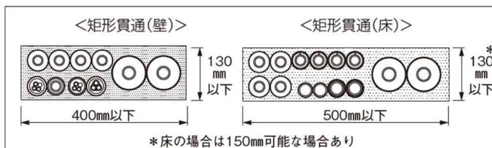
図-20 矩形貫通の場合
