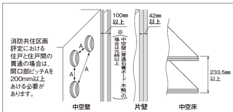
図-27 貫通開口部の設定
