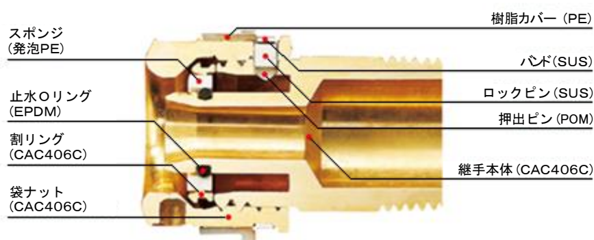
図－10 パーフェクトロックの構造
