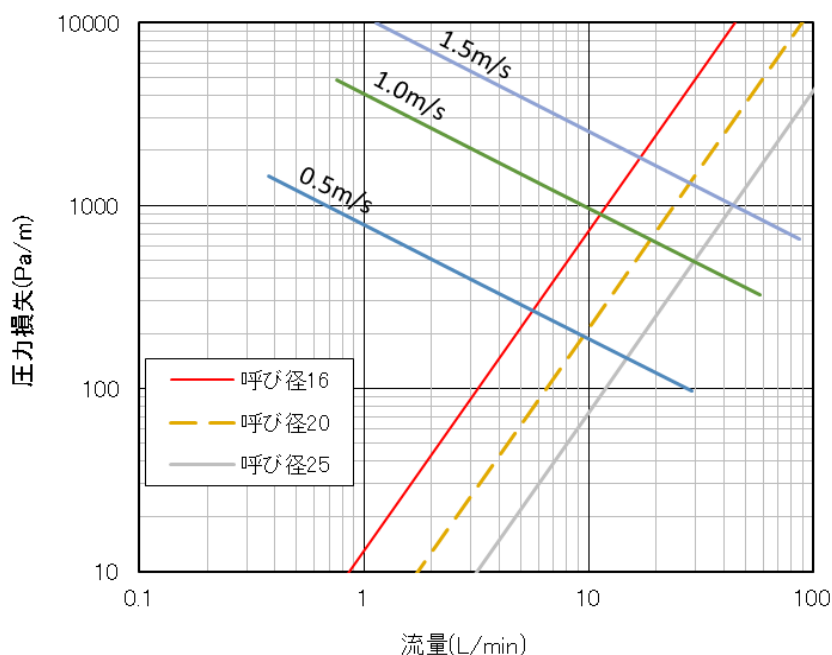
図-16 マルチ 1 パイプの流量線図
