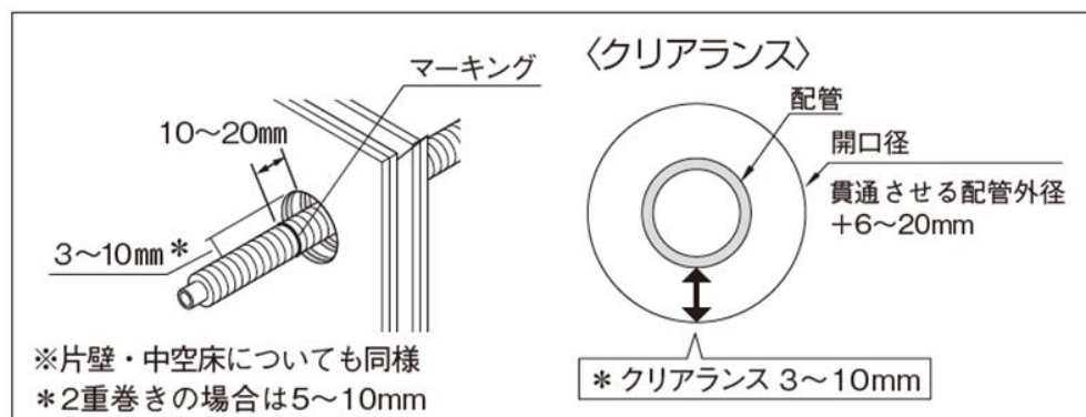
図-28 配管の設置(中空壁・片壁・中空床共通)
