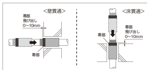
図－25 耐火プラグのスライド
