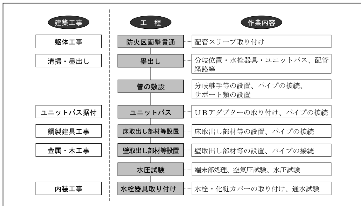
図４－１６ 分岐工法施工フローチャート
