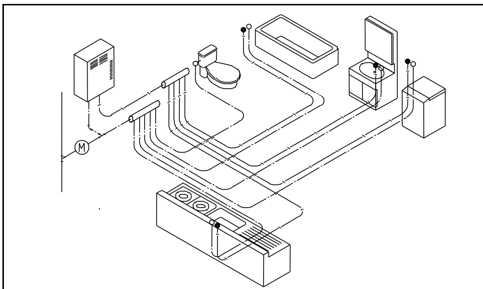
図１－２ ヘッダー工法概略図
