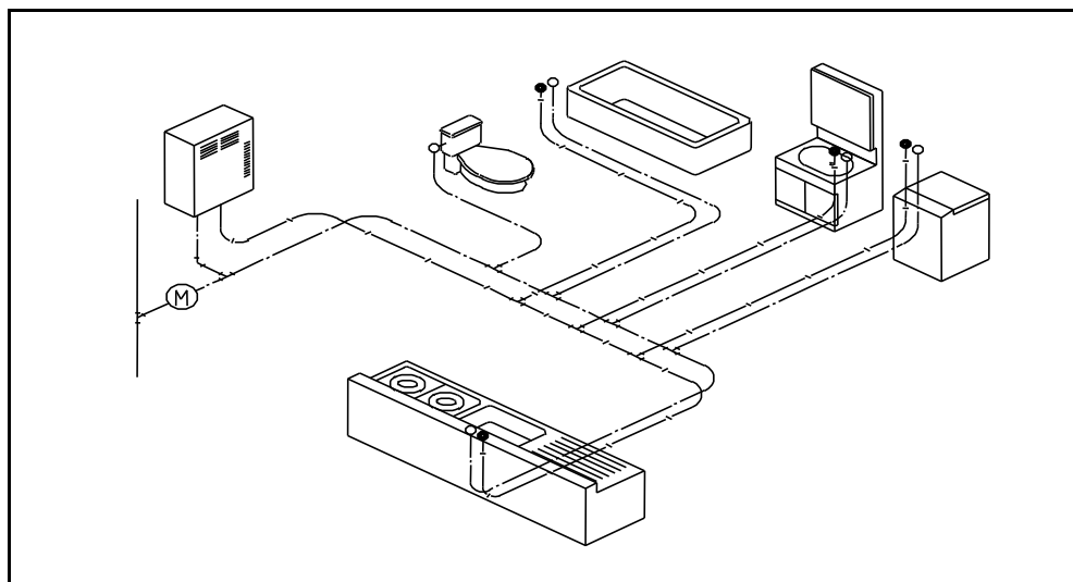
図１－１ 分岐工法概略図
