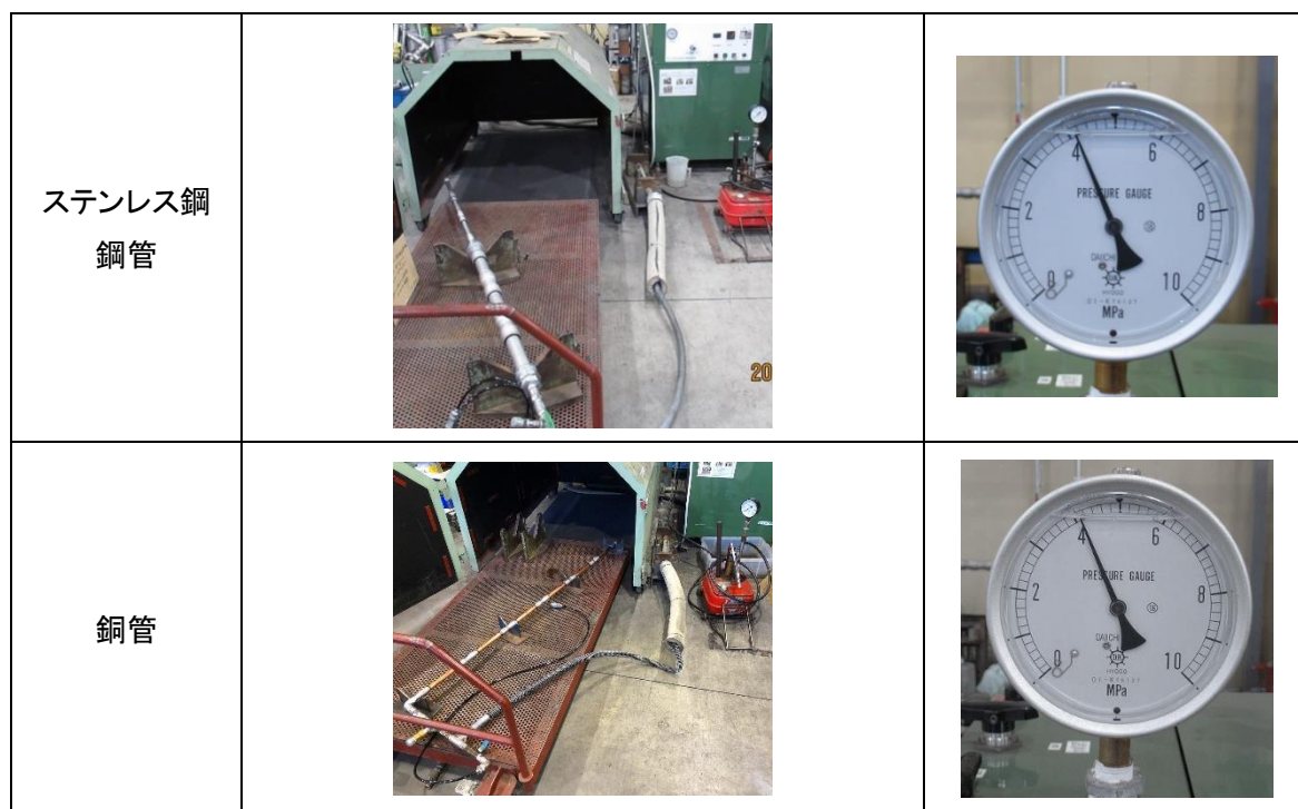
写真 4-6 内圧繰返し試験写真
