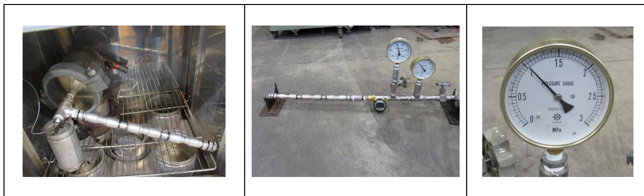
写真 4-9 実体による促進劣化試験写真
