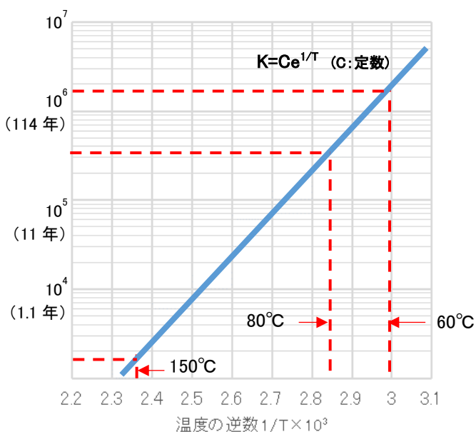
図4-12 温度と寿命時間との関係
