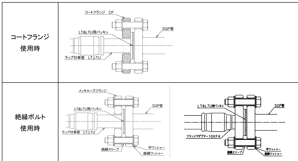
図 5-3-1 フランジによる接合
