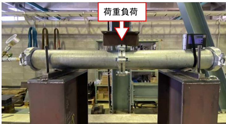
写真 6-4-1 曲げ試験外観
