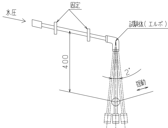
図 4-14 揺動試験
