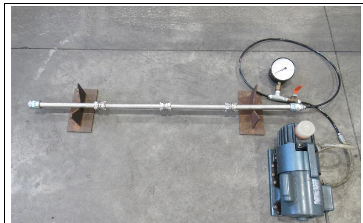
写真 4-2 負圧試験
