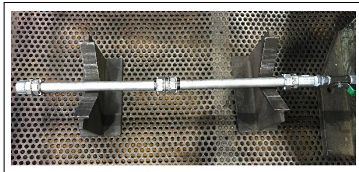
写真 4-3 水圧試験
