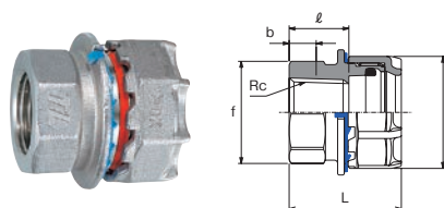
めすアダプター (AQ)
