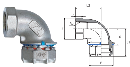
めすアダプターエルボ (AQL)
