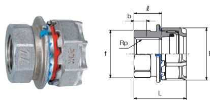
給水栓用ソケット (WS)
