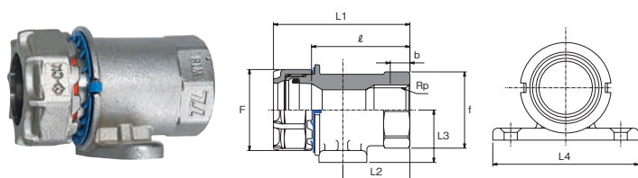
給水栓用座付ソケット (WTS)
