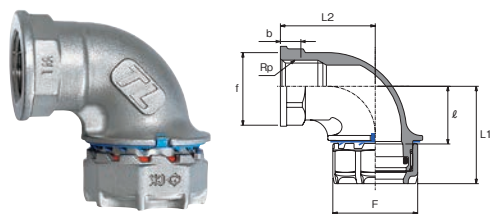
給水栓用エルボ (WL)
