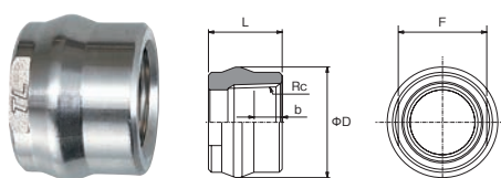
ブッシング (Bu)
