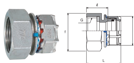
メーターソケット (MS)
