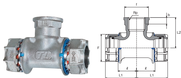
給水栓用チーズ (WT)
