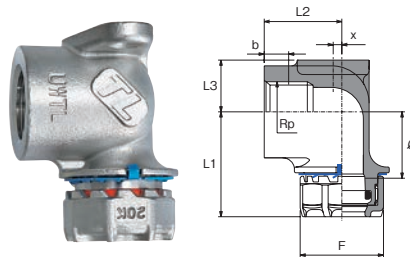
上取型給水栓用座付エルボ (UWTL)
