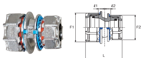
径違いソケット (RS)
