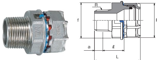
おすアダプター (AP)
