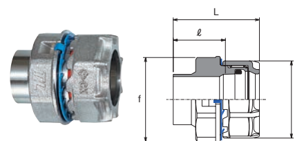
溶接アダプター (YA)
