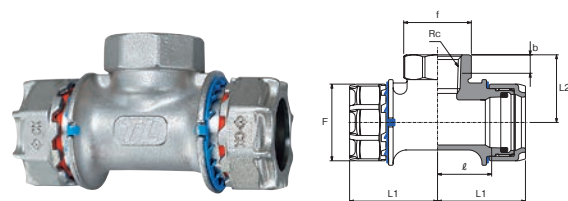
径違いチーズ枝部ねじ (RTQ)
