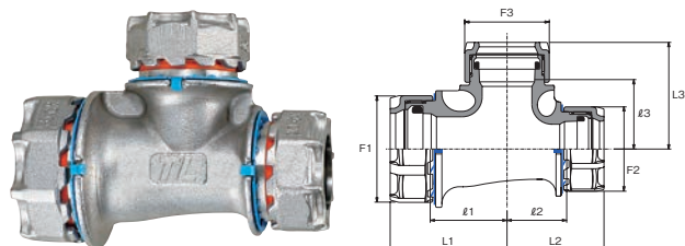
三方径違いチーズ (RT)
