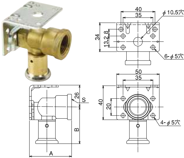
両座付アダプターエルボ○
