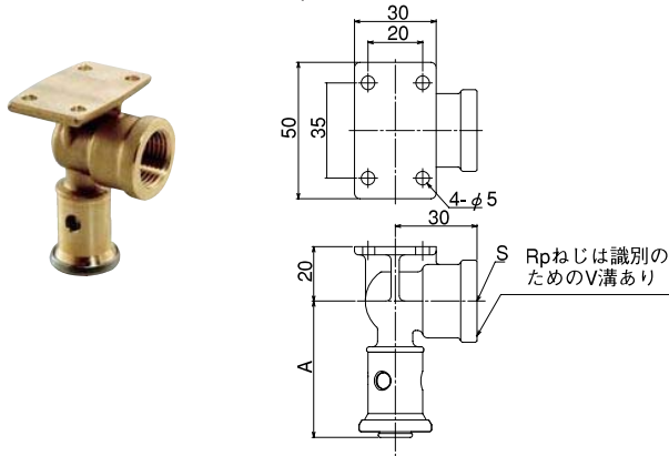
上座付アダプターエルボ o
