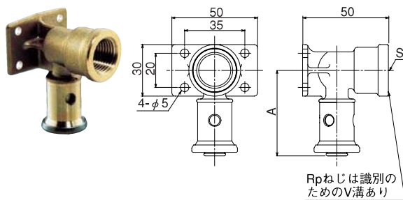
座付給水栓エルボ o (Rpねじ)
